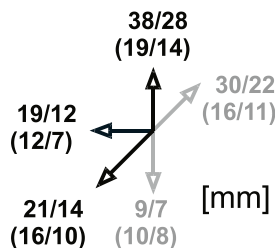
Figur 3: Orienteringsdetekteringsafstand - aktivering/deaktivering på en ikke-magnetisk (magnetisk) overflade
