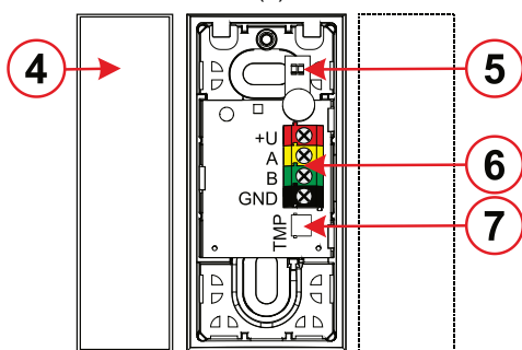
Figur 2: Beskrivelse af detektorens indvendige dele: 4 - permanent magnet; 5 - LED-indikatorer; 6 - busklemmen; 7 - sabotagekontakt
