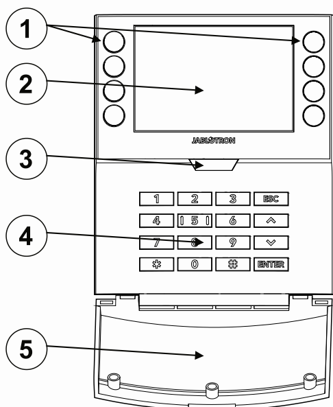
Obr. 1: 1 – ovládací tlačítka; 2 – LCD displej; 3 – systémový indikátor/tlačítko; 4 – klávesnice s RFID čtečkou; 5 – kryt;
