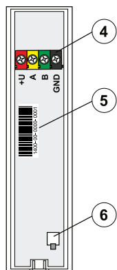
Obrázek: 1 – místo pro aretační šroubek, 2 – západka pro otevření, 3 – indikační LED, 4 – svorky sběrnice, 5 – sériové číslo, 6 – ochranný kontakt krytu
