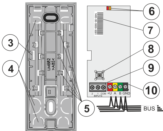
Afbeelding 2: 3 – PCB-tab; 4 – uitsparingen; 5 – bevestigingsklemmen voor kabels die uit de bovenste uitsparingen leiden; 6 – rode en gele LED-indicator; 7 – productiecode; 8 – sabotagesensor; 9 – klem van magnetische detectoren; 10 – busklem;
