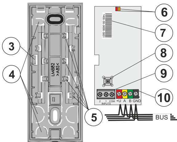
2. ábra: 3 – a nyomtatott áramkört lap rögzítő nyelve; 4 – kiterjesztő kábelerőszívő nyílások; 5 – kábelerőszívő fűlek; 6 – piros és sárga LED visszajelzők; 7 – gyártási sorozatszám; 8 – szabotázs kontaktus; 9 – a külső érzékelők sorcsatlakozói; 10 – az adatbusz sorcsatlakozói
