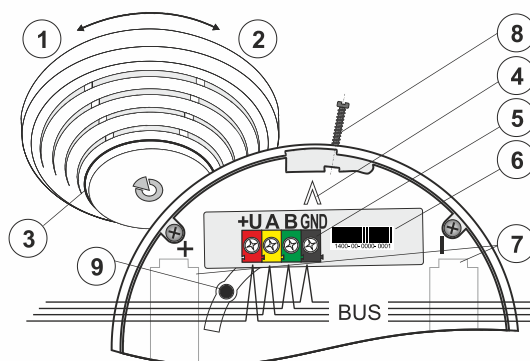
obrázek 6: 1 – uvolnění detektoru; 2 – upevnění detektoru; 3 – optická signalizace stavu; 4 – orientační šipka pro nasazení; 5 – svorkovnice sběrnice; 6 – sériové číslo; 7 – prostor pro vložení baterií; 8 – aretační šroub; 9 – tlačítko pro spuštění testu;
