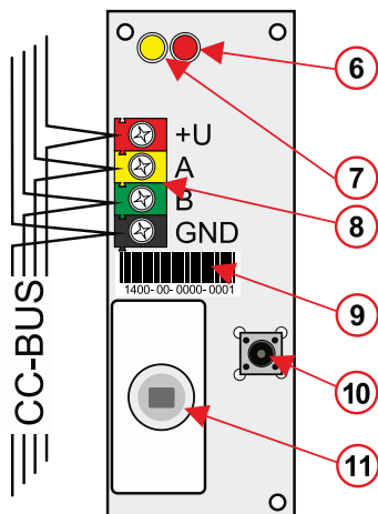
Obrázek 2.: 6 – červený LED indikátor – aktivace; 7 – žlutý LED indikátor – porucha; 8 – svorky sběrnice; 9 – sériové číslo; 10 – sabotážní spínač krytu; 11 – PIR senzor
