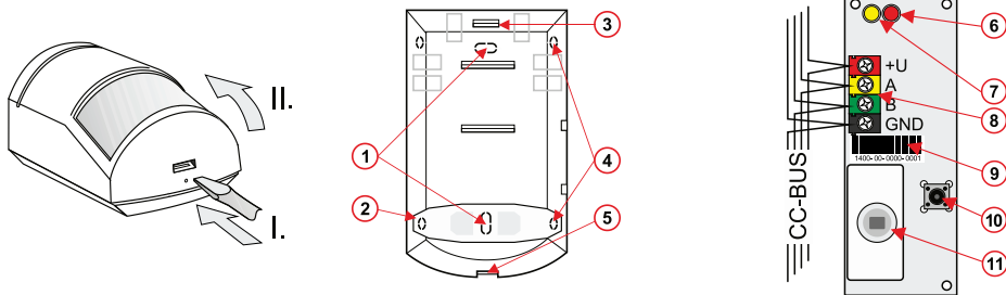
Obrázok 1: Popis vonkajších a vnútorných častí výrobku
