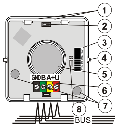
Obr. 2: 1 – kontrolky; 2 – vnútorné tlačidlá; 3 – sériové číslo; 4 – čipy držiaka; 5 – piezoelektrická siréna; 6 – svorkovnica zbernice; 7 – sabotážne kontakty; 8 – konektor pre pripojenie akumulátora;
