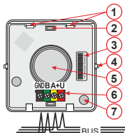
Obr. 2: Popis vnitřních částí sirény
