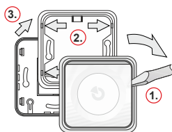
Obr. 1: Demontáž sirény před instalací
