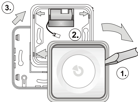
Obr. 1 – Demontáž sirény pred inštaláciou
