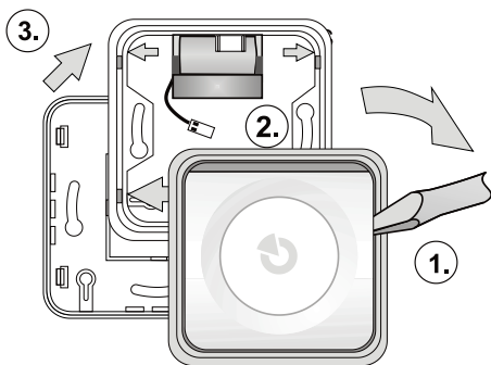
Figura 1: desmontagem da sirene antes da instalação
