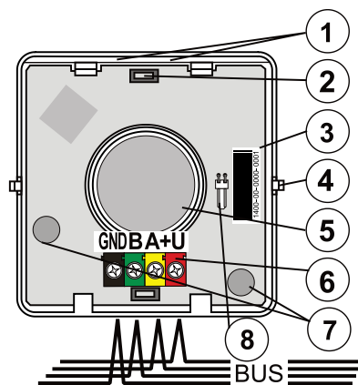
Figura 2: 1 - indicadores LED; 2 - botões; 3 - código de produção; 4 - patilhas da peça com botões; 5 - sirene piezoelétrica; 6 - terminal BUS; 7 - sensores de tampo; 8 - conector da bateria para BAT-3V2-CR2
