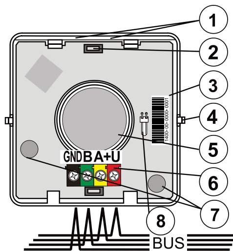
Afbeelding 2: 1 – LED-indicatoren; 2 – knoppen; 3 – productienummer; 4 – knop tabs; 5 – piezo-elektrische sirene; 6 – busklem; 7 – sabotagesensoren; 8 – batterijconnector voor BAT-3V2-CR2
