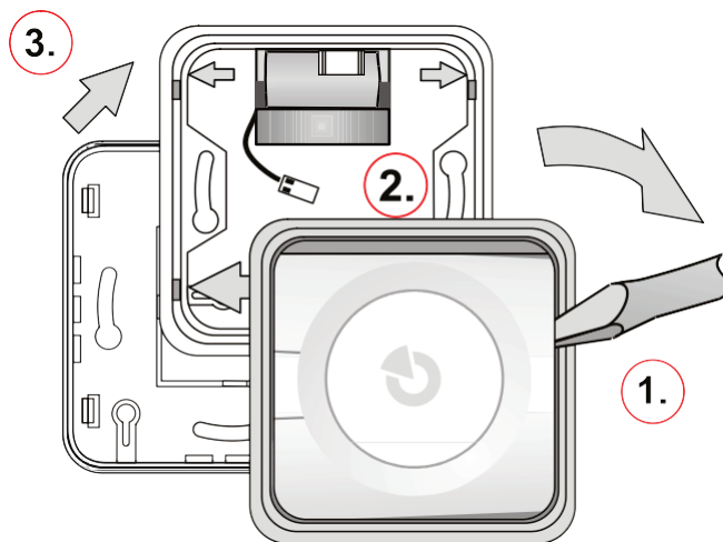
Billede 1: Afmontering af sirenen før installation
