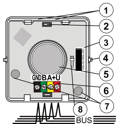
Figure 2 : 1 - Voyants LED ; 2 - Touches ; 3 - Numéro de production ; 4 - Languettes de la touche ; 5 - Sirène piézo-électrique ; 6 - Borne du BUS ; 7 - Capteurs de sabotage ; 8 - Connecteur de la batterie pour BAT-3V2-CR2
