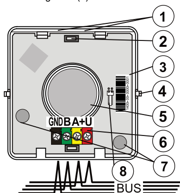
obr. 2: 1 – LED signálka; 2 – vnitřní tlačítka; 3 – sériové číslo; 4 – čepy hmatníku; 5 – piezoelektrická siréna; 6 – svorky sběrnice; 7 – senzory sabotáže; 8 – konektor pro připojení akumulátoru BAT-3V2-CR2
