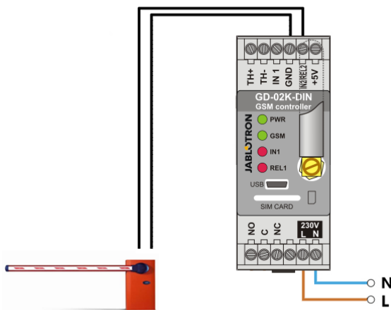
Obr. 2 Použití GD-02K-DIN pro ovládání závoř.
