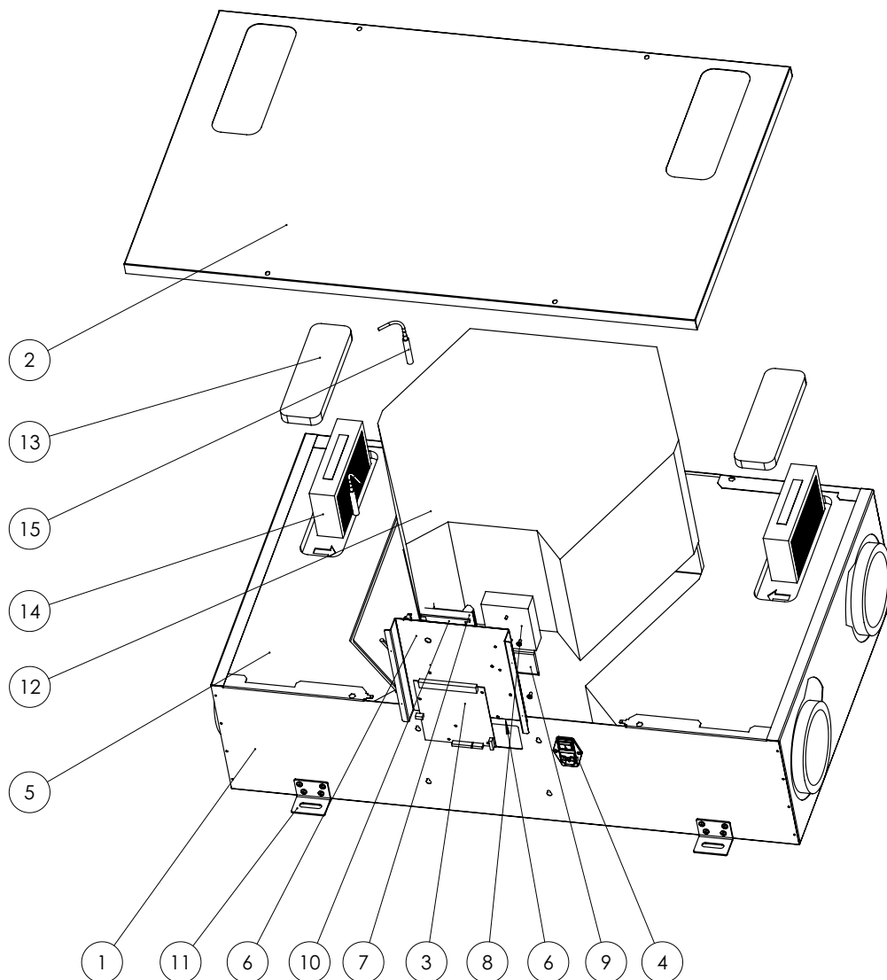
Obrázek 3 – Konstrukční části
